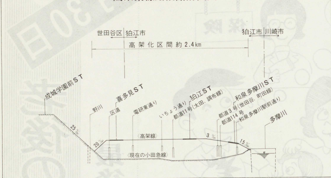
高架案線路縦断計画図
